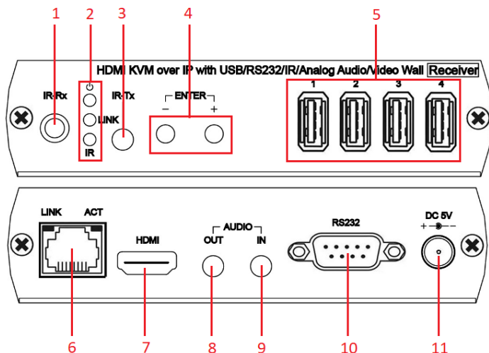
Рис.6 Приемник НКМ02БР. Разъемы, кнопки и индикаторы передней и задней панелей
